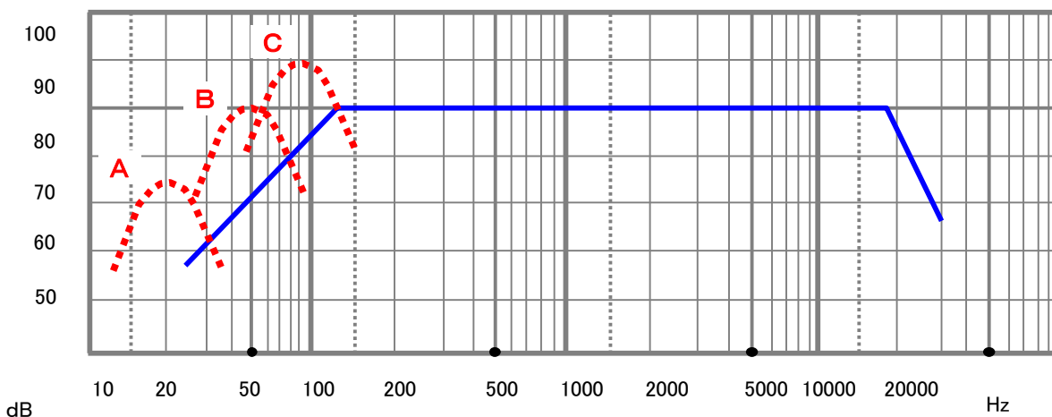
周波数特性グラフ(参考図)
